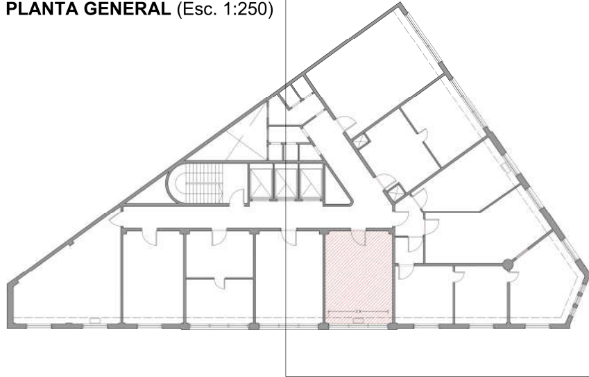
PLANTA 4° PISO (2) (Esc. 1:150)
